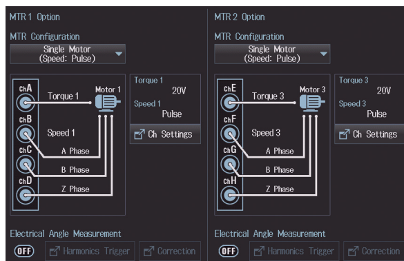
Для одновременного измерения 4 двигателей используйте совместно опции /MTR1 и /MTR2.
