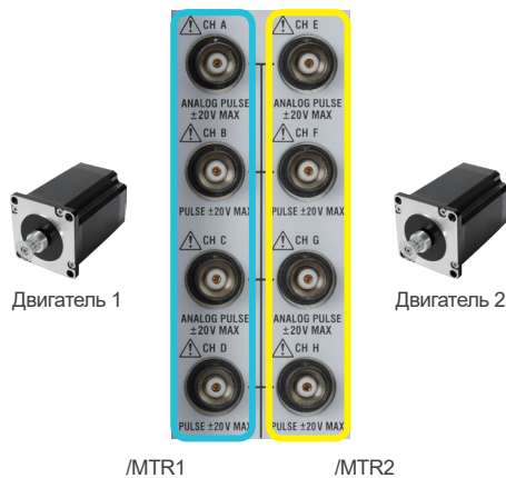
Один WT5000, сконфигурированный для одновременных синхронизированных измерений от 2 двигателей, для определения крутящего момента, скорости вращения, направления и электрических углов фаз A/B и Z
