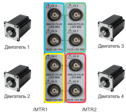
Один WT5000, сконфигурированный для одновременных синхронизированных измерений с 4 датчиков крутящего момента и вращения, чтобы определить полный кпд 4 двигателей
