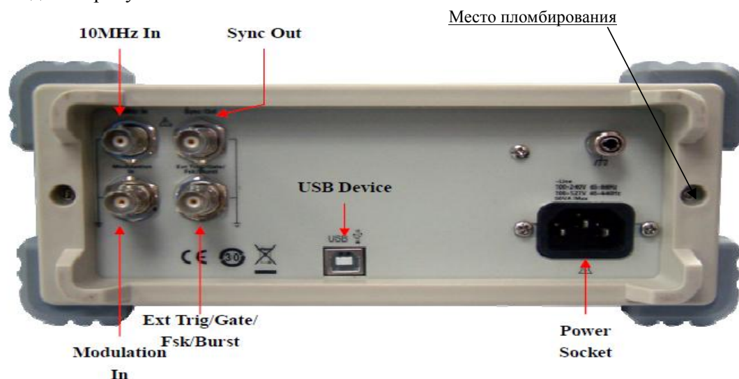
Рисунок 2 – Вид задней панели генератора
