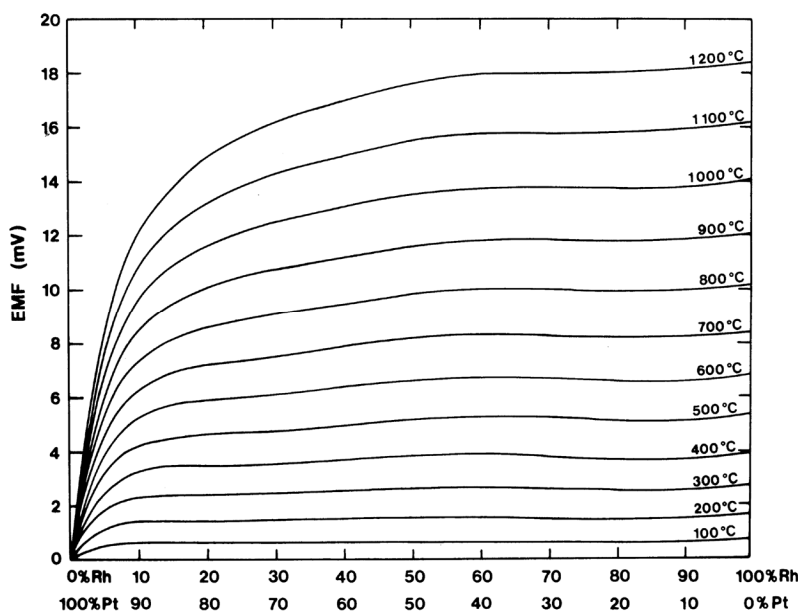
Рисунок 1. ЭДС родий-платиновых сплавов по сравнению с платиной
