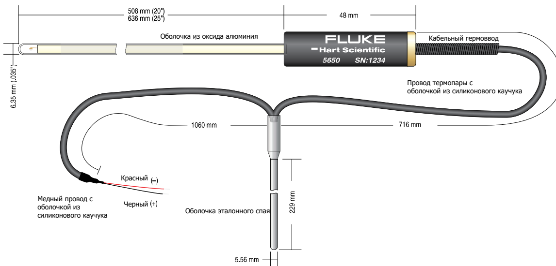
Рисунок 2. Конструкция и стандартные размеры
