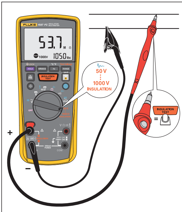
Рис. 9. Проверка сопротивления изоляции
