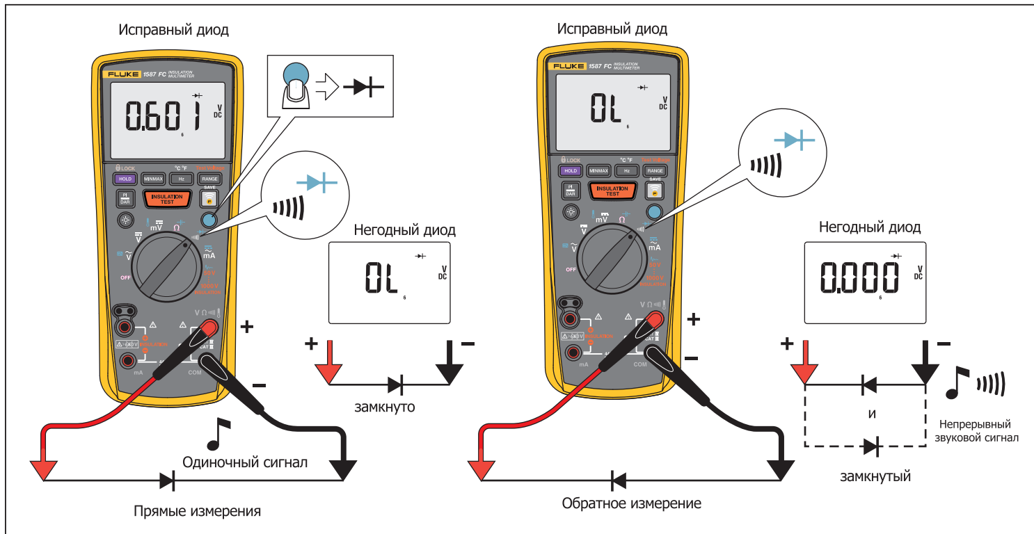
Рис. 7. Проверка диодов
