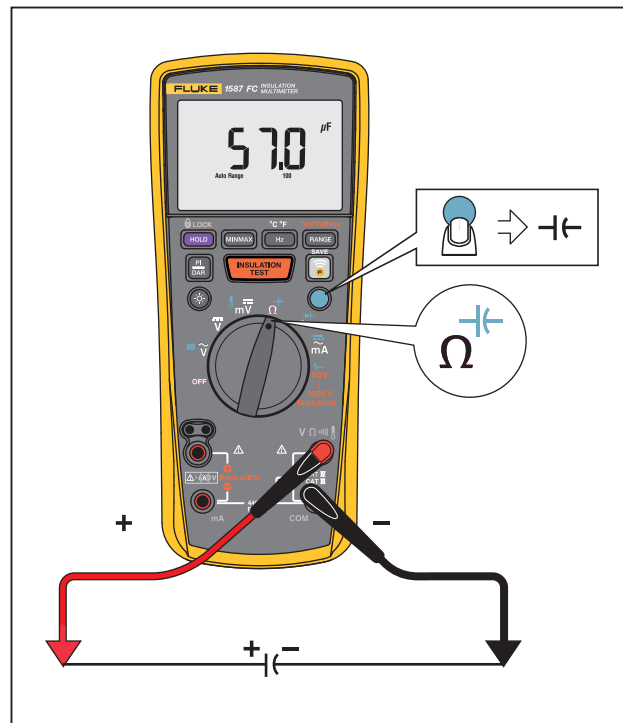
Рис. 5. Измерение емкости
