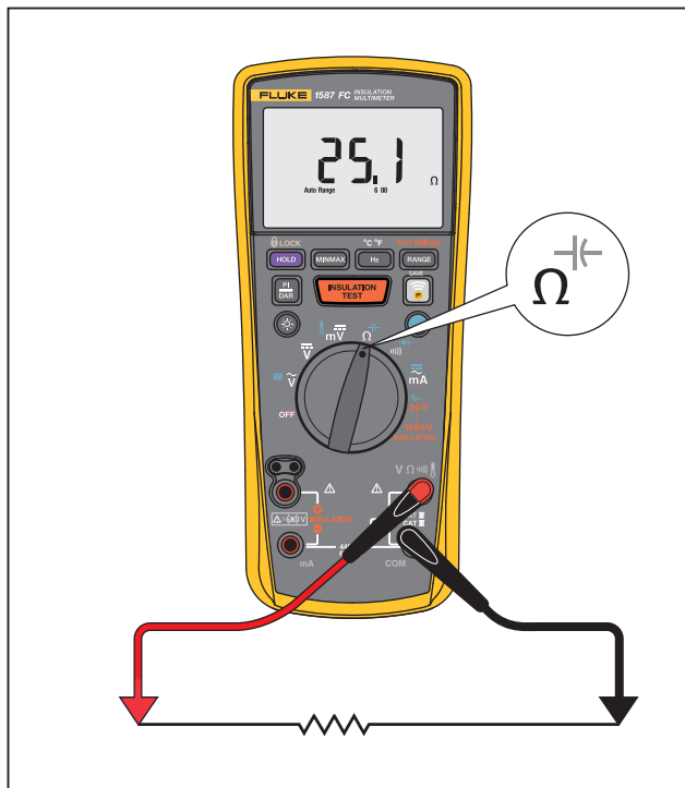
Рис. 4. Измерение сопротивления
