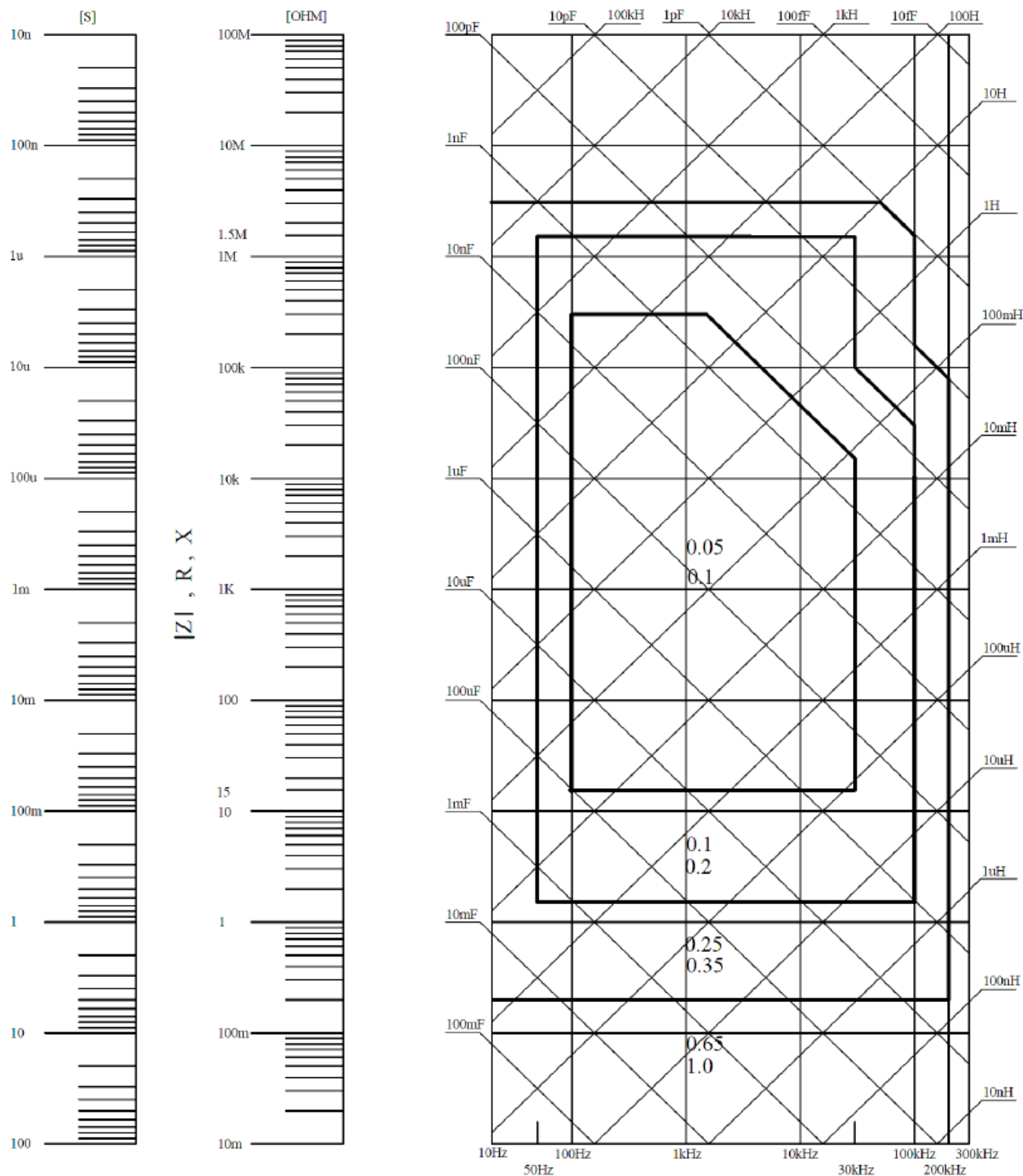
Рисунок 3 - Базовая погрешность A, где верхнее значение погрешности для режимов «Slow» и «Medium», нижнее - для «Fast»
