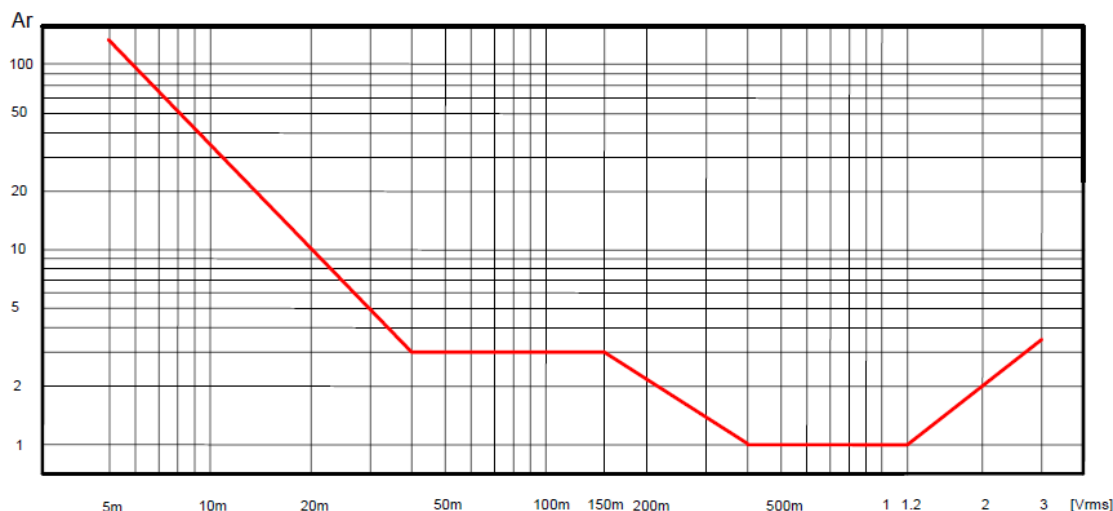
Рисунок 4 - Поправочный коэффициент A_T по уровню тест-сигнала (напряжению)
