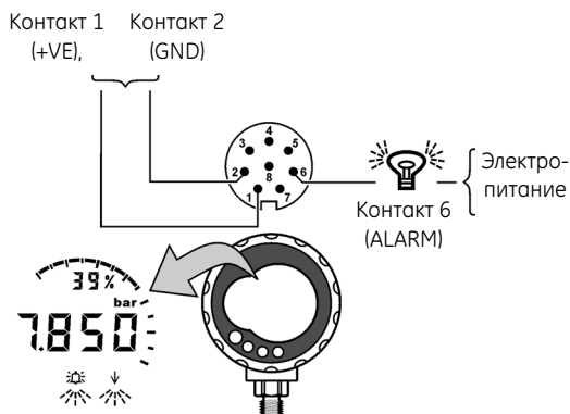
Рис. 3: Пример конфигурации — вывод сигнала
