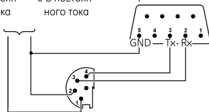
Рис. 4: Пример конфигурации: RS232
