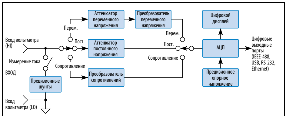
Рис. 1. Структурная схема цифрового мультиметра
