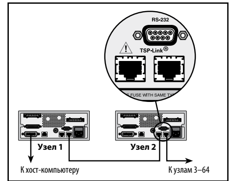
Рис. 10. Задняя панель приборов серии 2600B
