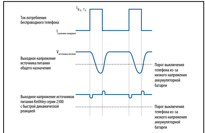
Рис. 3. Сравнение отклика на изменение нагрузки источника питания общего назначения и источника питания Keithley серии 2300 с быстрой динамической реакцией.
