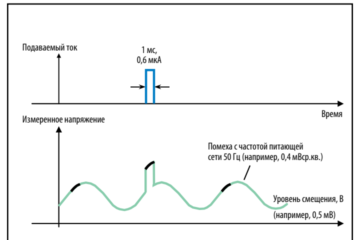
Рис. 7. При работе с низкими уровнями напряжения измерения могут быть подвержены помехам с частотой сети электропитания. Применение синхронизации с напряжением питающей сети устраняет помехи с частотами, кратными 50 Гц
