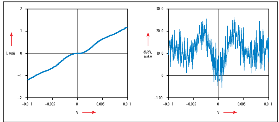
Рис. 9,а. Вольтамперная характеристика
