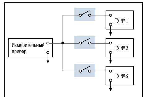
Рис. 4. Мультиплексор
