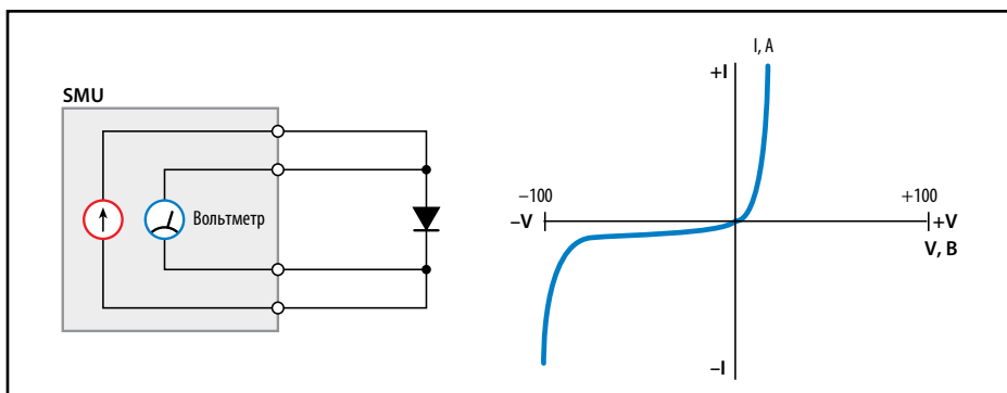
Рис. 5. Типовая вольтамперная характеристика диода
