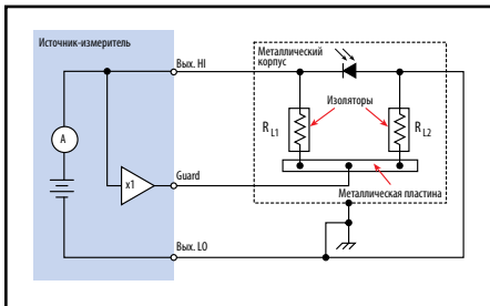
Рис. 8. Схема охранного экранирования поддерживает потенциал охранного электрода равным потенциалу электрода «Выход, высокий потенциал»
