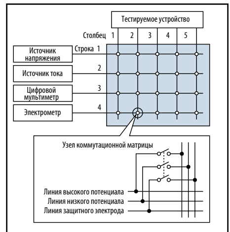
Рис. 3. Коммутационная матрица
