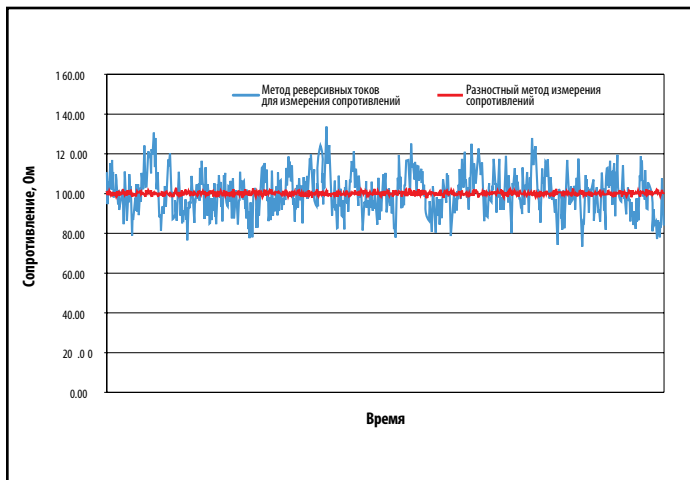
Рис. 6. Результаты измерения сопротивления резистора 100 Ом при токе источника 10 нА (1000 отсчетов полученных разными методами)
