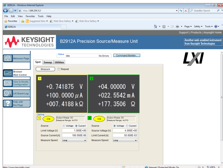
Рис.7. Графический веб-интерфейс
