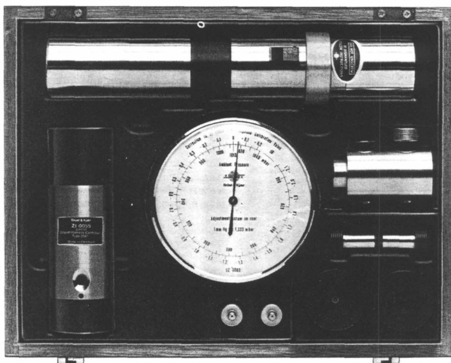
Рис. 1. Интенсиметрический калибратор 3541 в деревянном ящике
