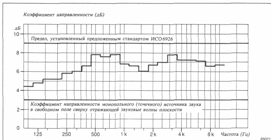
Рис. 2. Номинальная кривая коэффициента направленности прибора 4204 в вертикальной плоскости
