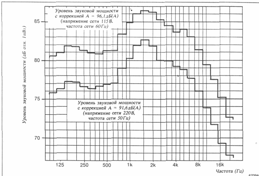
Рис. 1. Номинальные кривые третьоктавных спектров мощности излучаемого прибором 4204 звука
