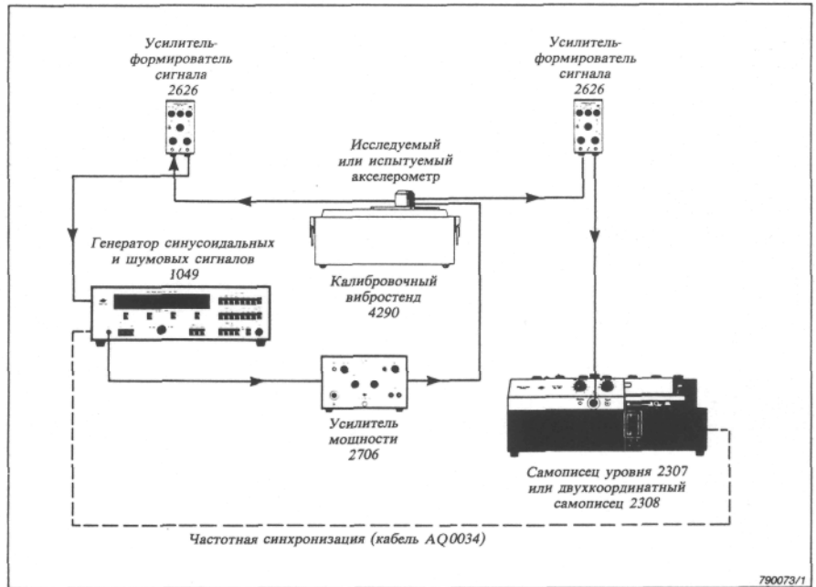
Рис. 1. Пример системы для автоматической регистрации амплитудно-частотных характеристик акселерометров
