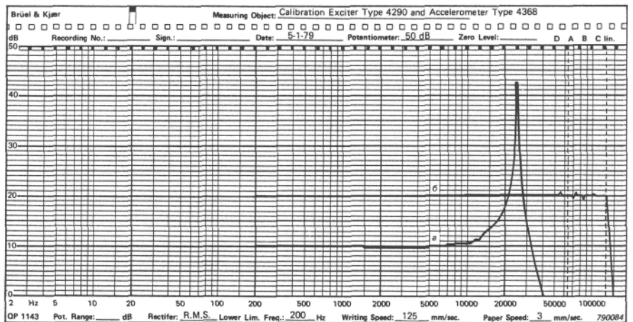
Рис. 2. Кривые, зарегистрированные показанной на рис. 1 автоматической системой: а. амплитудно-частотная характеристика акселерометра б. частотная зависимость ускорения стола вибростенда 4290
