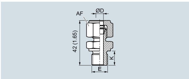
Компрессионный фитинг, размеры в мм (дюймах)
