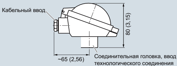
Соединительная головка, алюминий, тип BV0, размеры в мм (дюймах)
