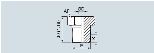
Припаяваемый штуцер NPT, размеры в мм (дюймах)
