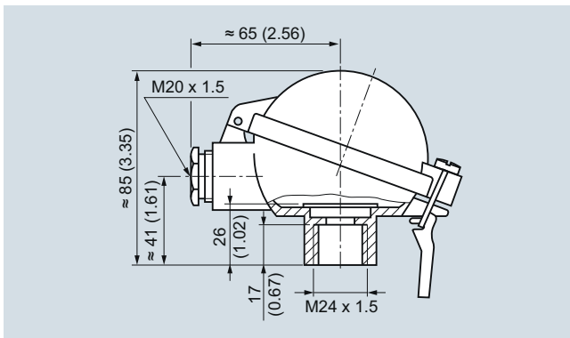
Соединительная головка, тип В, степень защиты IP65, из литого легкого сплава, со стандартной откидной крышкой, размеры в мм (дюймах)
