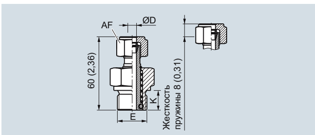
Подпружиненный компрессионный фитинг, размеры в мм (дюймах)
