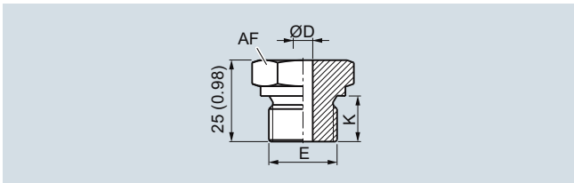
Припаяваемый штуцер, метрический, размеры в мм (дюймах)
