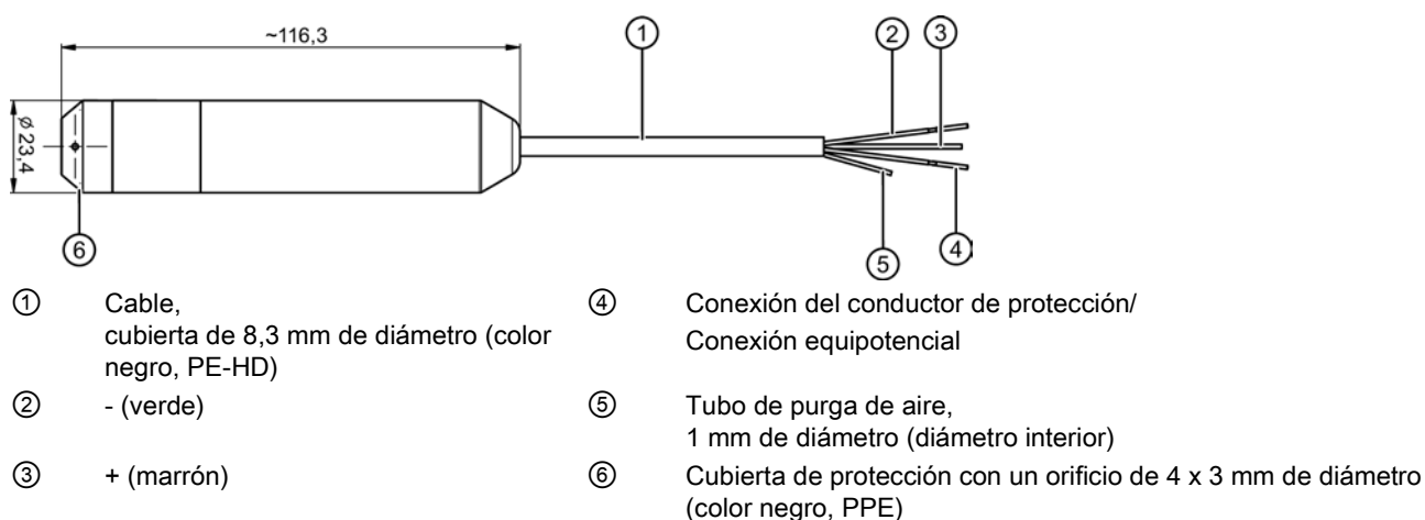
Figura 9-1 Transmisor de presión, dimensiones en mm
