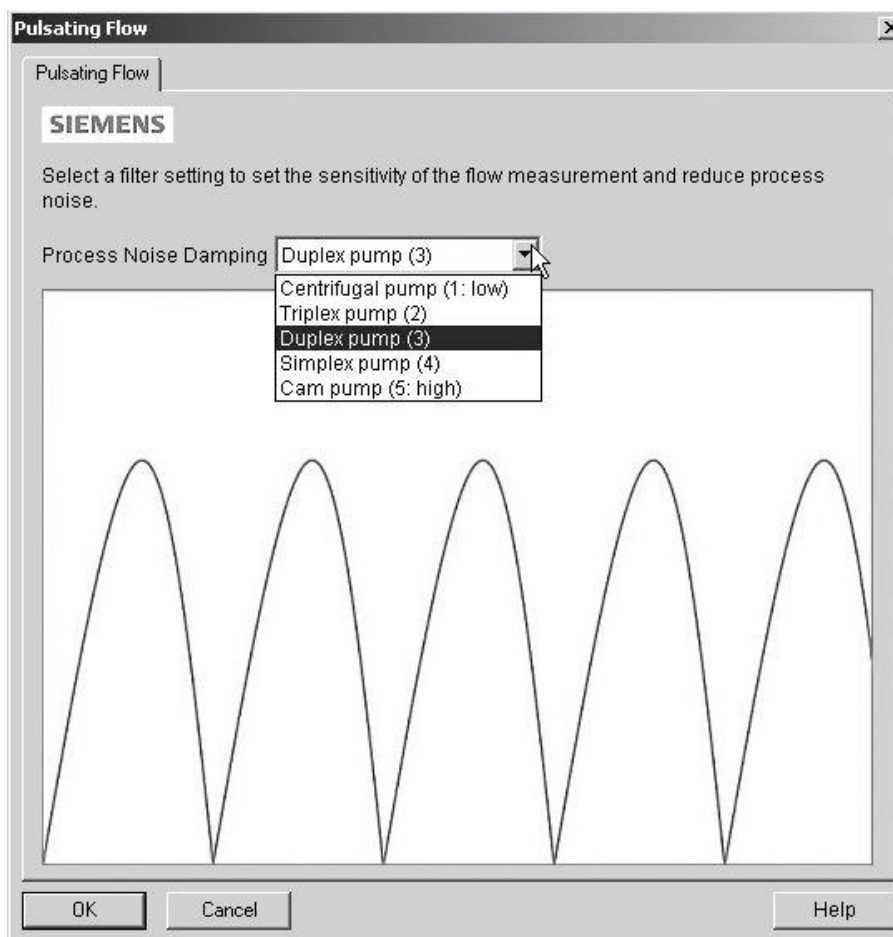
Рис. 6-8. Настройка фильтра
