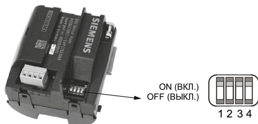
Рис. 5-3. Расположение DIP-переключателей [все установлены в положение ON (Включено)]
