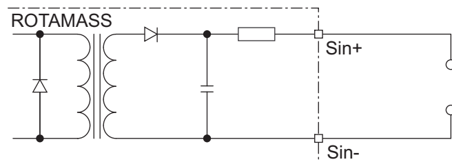
Рис. 39. Соединение входа состояния
